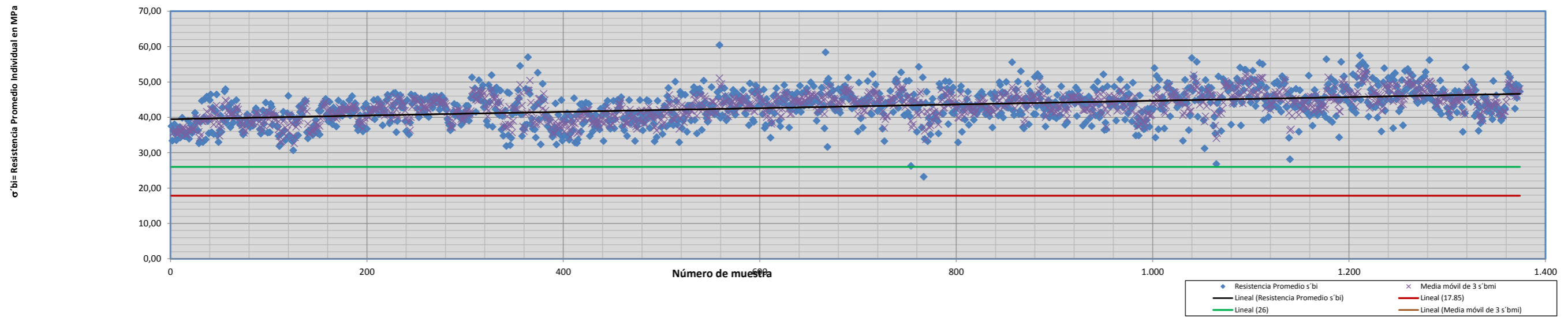
Gráfico de dispersión - Lomax Resultados a 28 días FC 400
